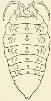
FIG. 35.— SYNIDOTEA TUBERCULATA . × 2½.
